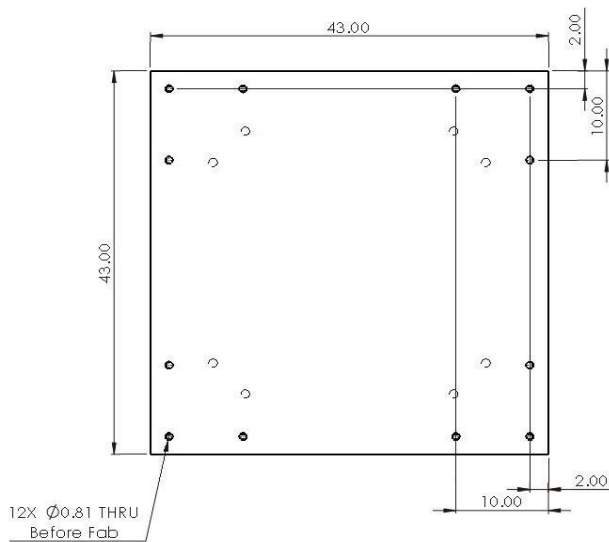
Robo Sawjet pedestal footprint
